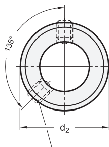
Druhý upínací šroub pro velikost d_1 = 80
